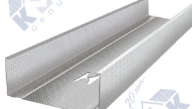
Профиль стоечный ПС 100*50
