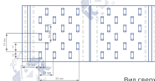
Вид сверху
